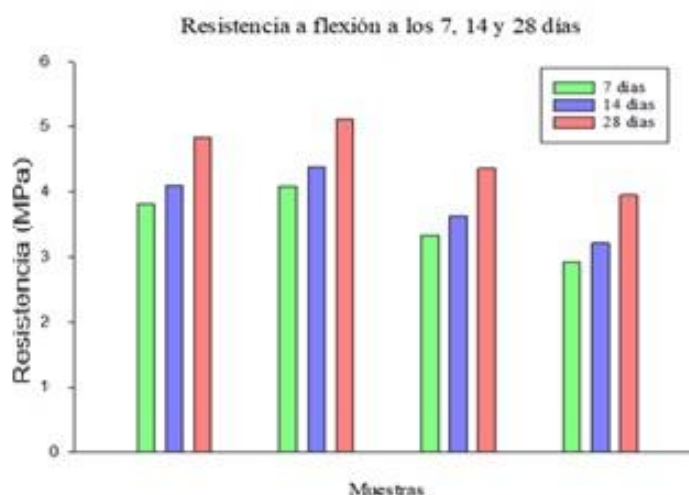
Figura 4. Resistencia a flexión a 7, 14 y 28 días de maduración con y sin CM. Fuente: los autores
