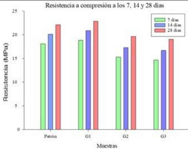
Figura 3. Resistencia a compresión a 7, 14 y 28 días de maduración con y sin CM. Fuente: los autores
