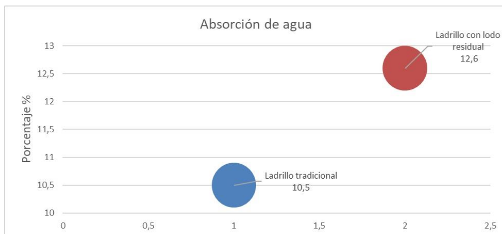
Figura 7. Absorción de agua. Fuente: los autores
