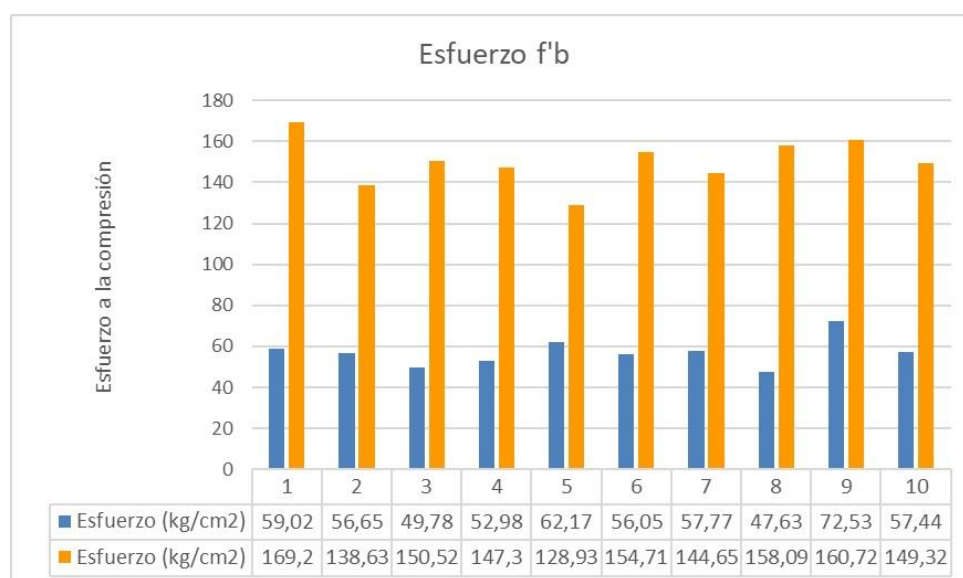
Figura 3. Resistencia a la compresión. Fuente: los autores
