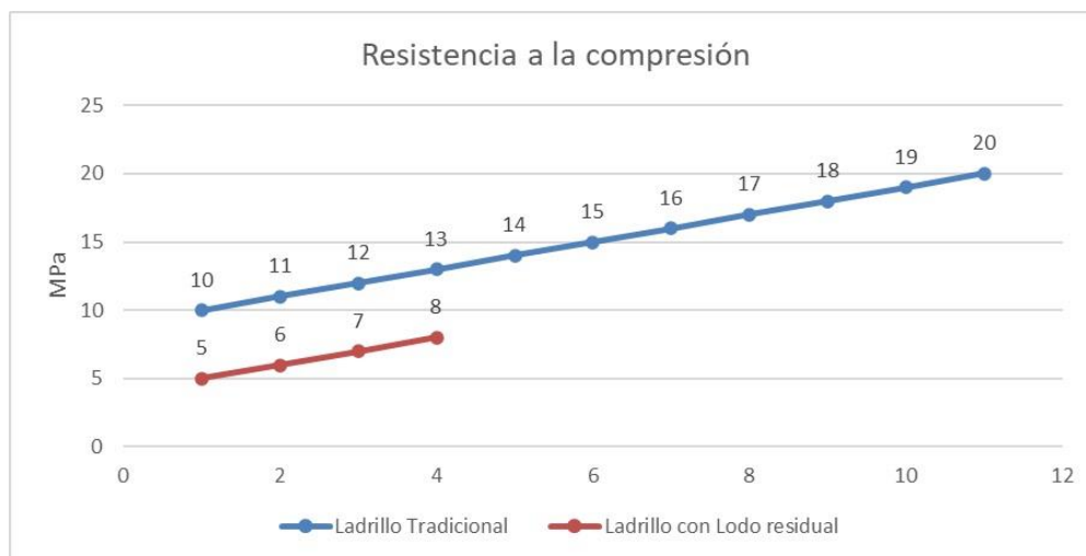
Figura 5. Resistencia a la compresión. Fuente: los autores
