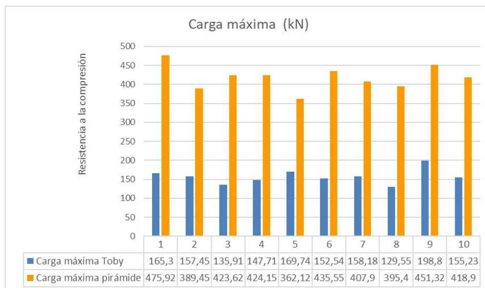
Figura 2. Cargas máximas soportadas. Fuente: los autores
