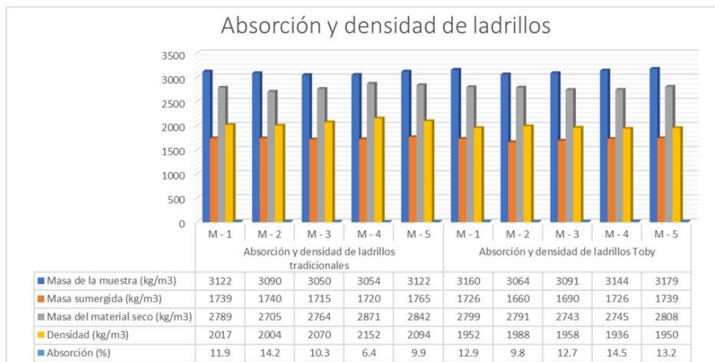
Figura 4. Absorción y densidad de ladrillos. Fuente: los autores
